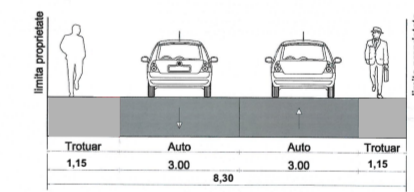
PROFIL STRADAL TRANSVERSAL STR. M. SADOVEANU - 8,30 m
