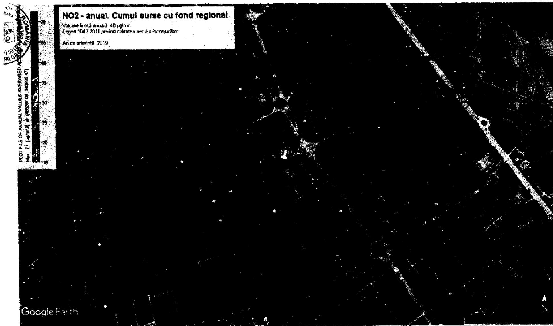
Figura nr. 2-11 Harta dispersie cumul surse cu fond regional – indicator NO 2 , concentrație medie anuală, an referință 2019, stația de monitorizare HD-1
