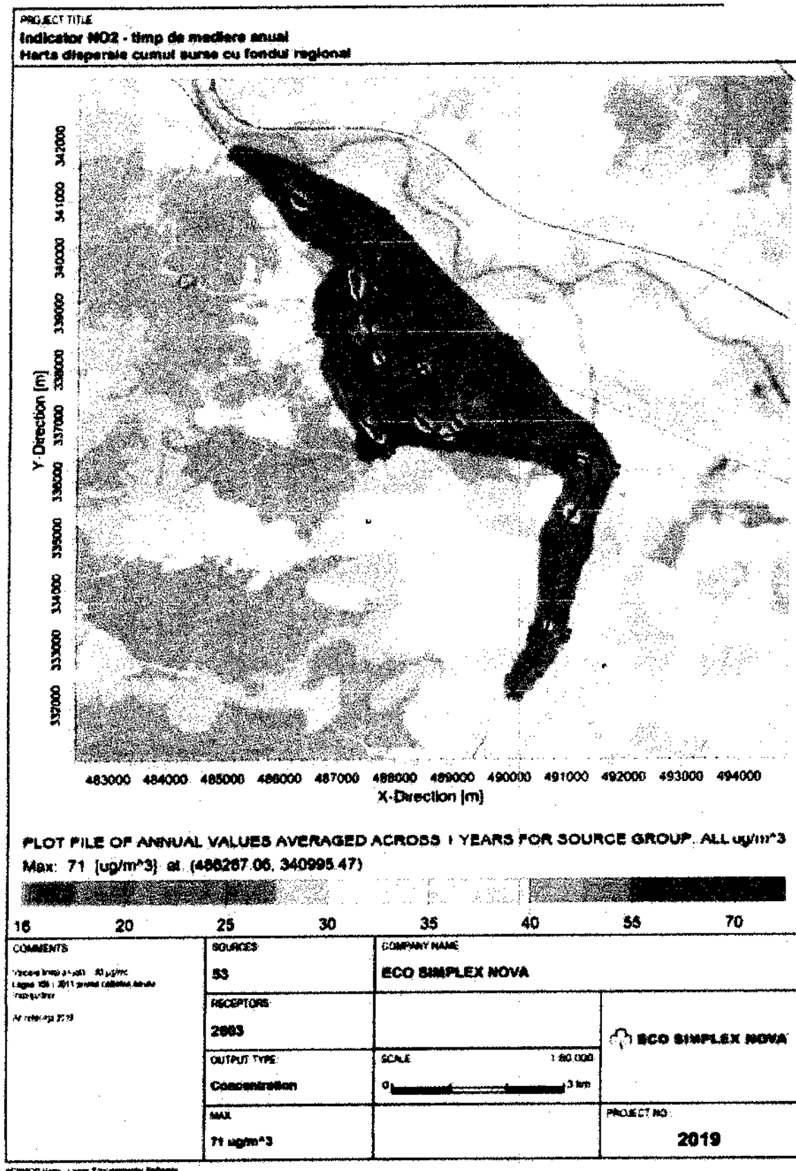
Figura nr. 2-12 Harta dispersie cumul surse cu fond regional – indicator NO 2 , concentrație medie anuală, an referință 2019, municipiul Deva
