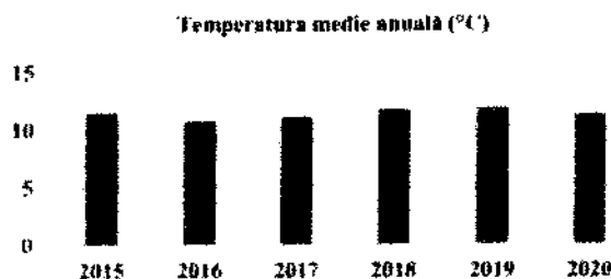
Figura nr. 2-14 Temperatura medie anuală
