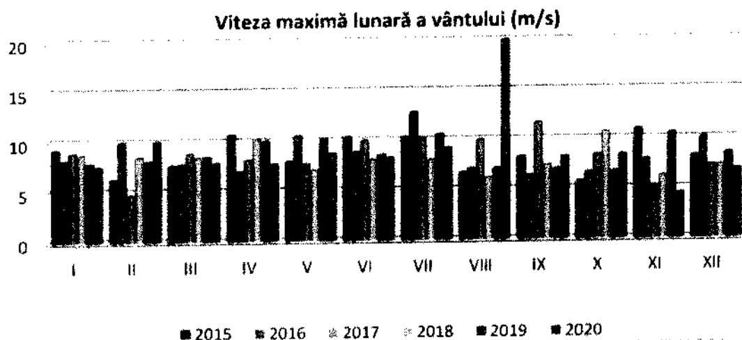
Figura nr. 2-27 Viteza maximă lunară a vântului
