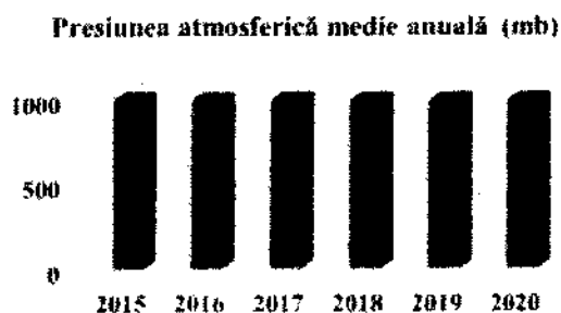
Figura nr. 2-21 Presiunea atmosferică medie anuală
