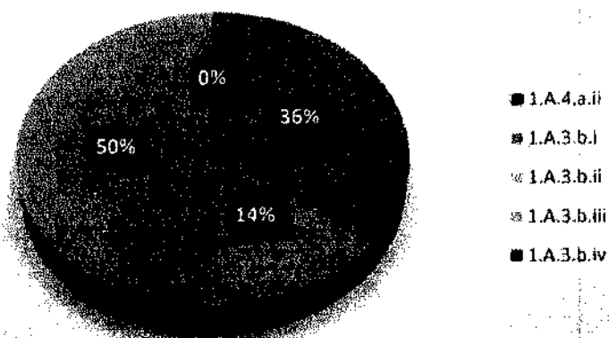
Figura nr. 4-4 Ponderea emisiilor de NO x din transport rutier și nerutier în anul de referință 2019
