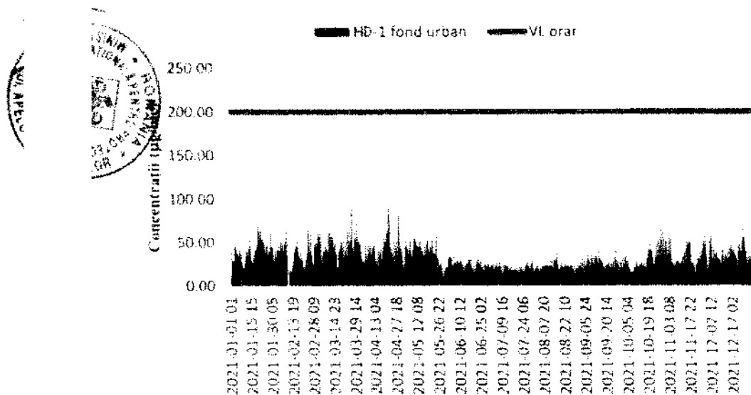
Figura nr. 3-5 Concentrații medii orare pentru dioxid de azot (NO 2 ) (µg/mc) înregistrate la stațiile automate de monitorizare din municipiul Deva, în anul 2021
