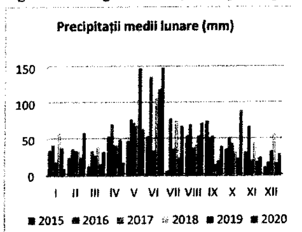
Figura nr. 2-23 Precipitații medii lunare
