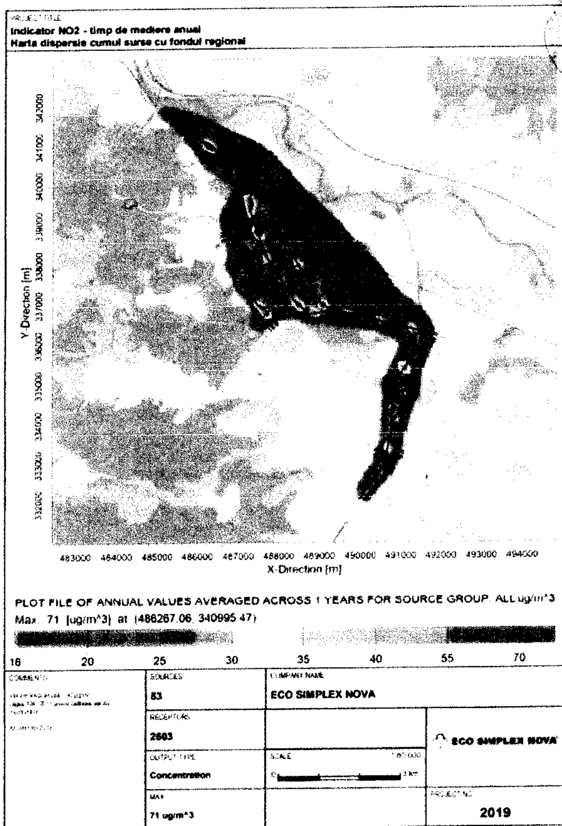
Figura nr. 4-10 Concentrația medie anuală pentru indicatorul NO 2 în municipiul Deva , în anul 2019
