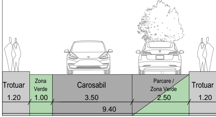
PROFIL TRANSVERSAL PROPUȘ D-D (9.40 M)
