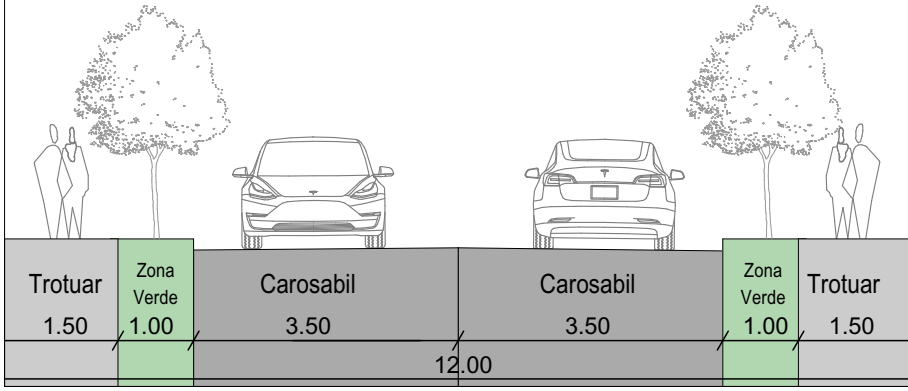
PROFIL TRANSVERSAL PROPUȘ E-E (12.00 M)
