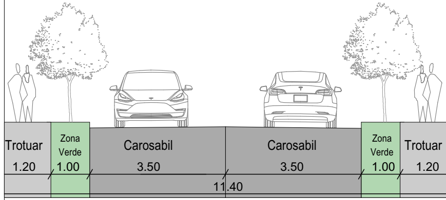
PROFIL TRANSVERSAL PROPUȘ C-C (11.40 M)
