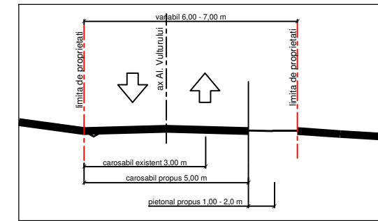
PROFIL STRADA Al. Vulturului
