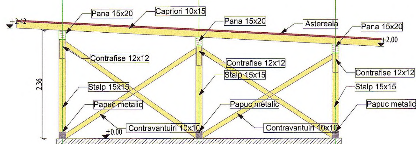
Sectiune sarpanta S01 1:50
