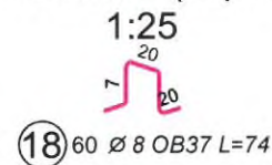
Distanțieri (capre)
