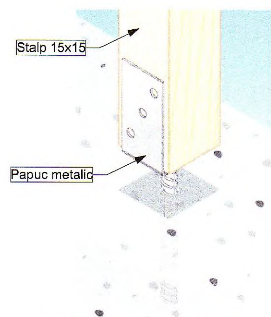
Detaliu imbinare baza stalp
