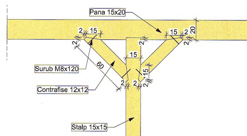
Detaliu imbinare stalp-pana
