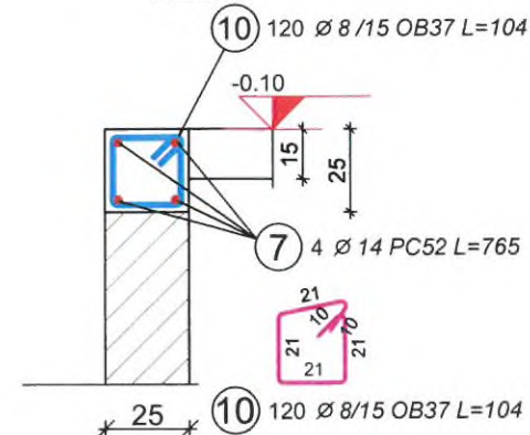
Centura b.a. 25x25 1:25
