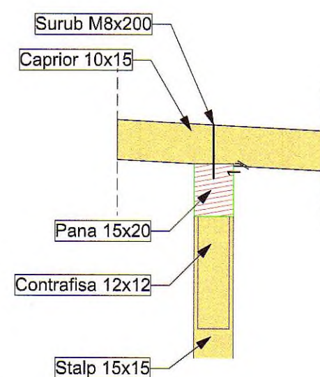
Detaliu imbinare caprior-pana
