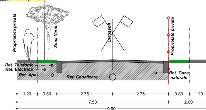
Profil transversal TIP B cu doua benzi de circulatie Propus
