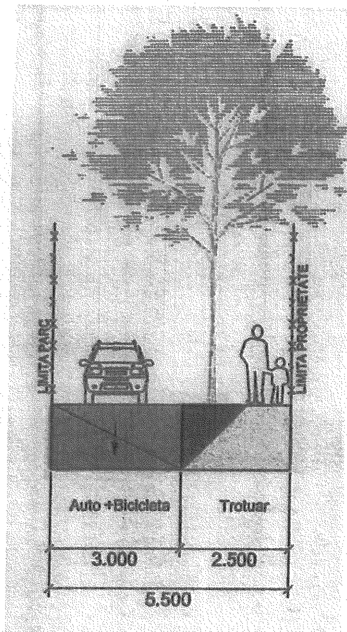
PROFIL STRADAL TRANSVERSAL TIP 6 – SENS UNIC – lățime 5,50 m
